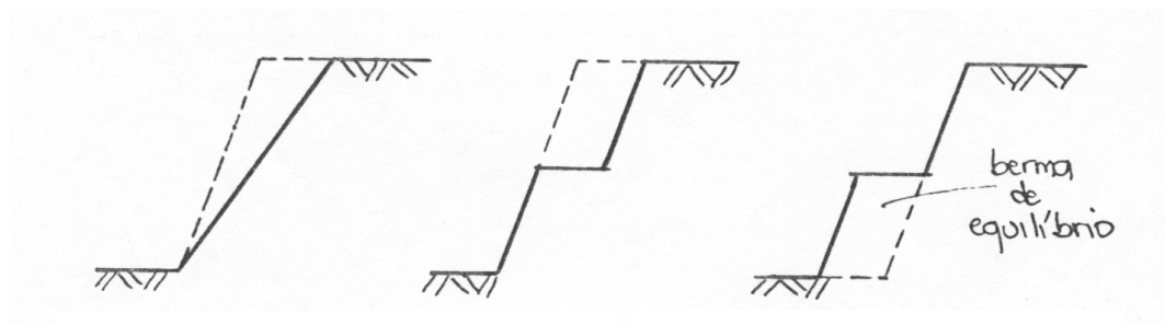
Figura 38- Estabilização de taludes através da alteração do ângulo de inclinação.
