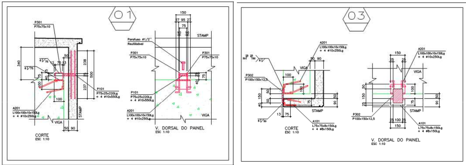
Sistema de Fixação De Gravidade ( 2X )
