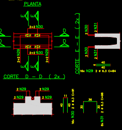
DETALHE "D" ( 2x )
