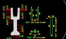
CORTE D - D
