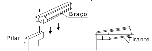
Encaixe Chumbadores - Apoio c/ Consolo
