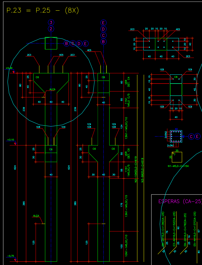
DETALHE I
